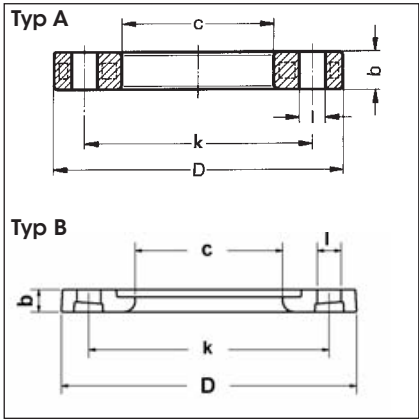
Flansch aus GGG, beschichtet, nach DIN 2501 für Vorschweißbunde PN 16 gebohrt
