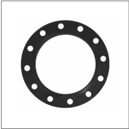
Flansch aus PP mit Stahleinlage, nach DIN 16962/16963 Teil 4 für Vorschweißbunde; PN 16 gebohrt
